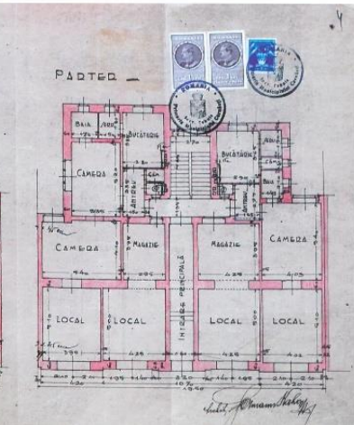
Житловий будинок на вул. Котляревського 14 Архітектор В. Грекул, 1937 р. ДАЧО 43/1/8684
