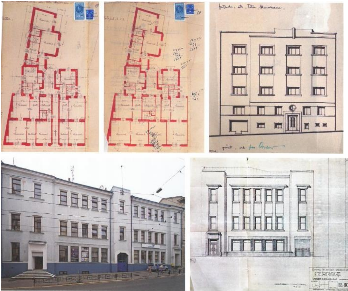
Будівля офісу пошти-телефону-телеграфу за вул. Університетська 3-5 Архітектор К. Нанеску, 1937 р. ДАЧО 43/1/7659
