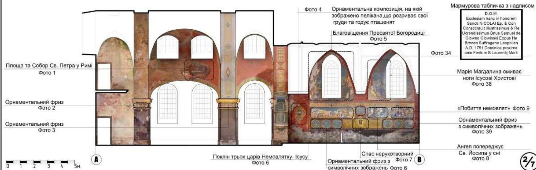
Розгортка по стіні А-В М 1:100 (існуючий стан)
