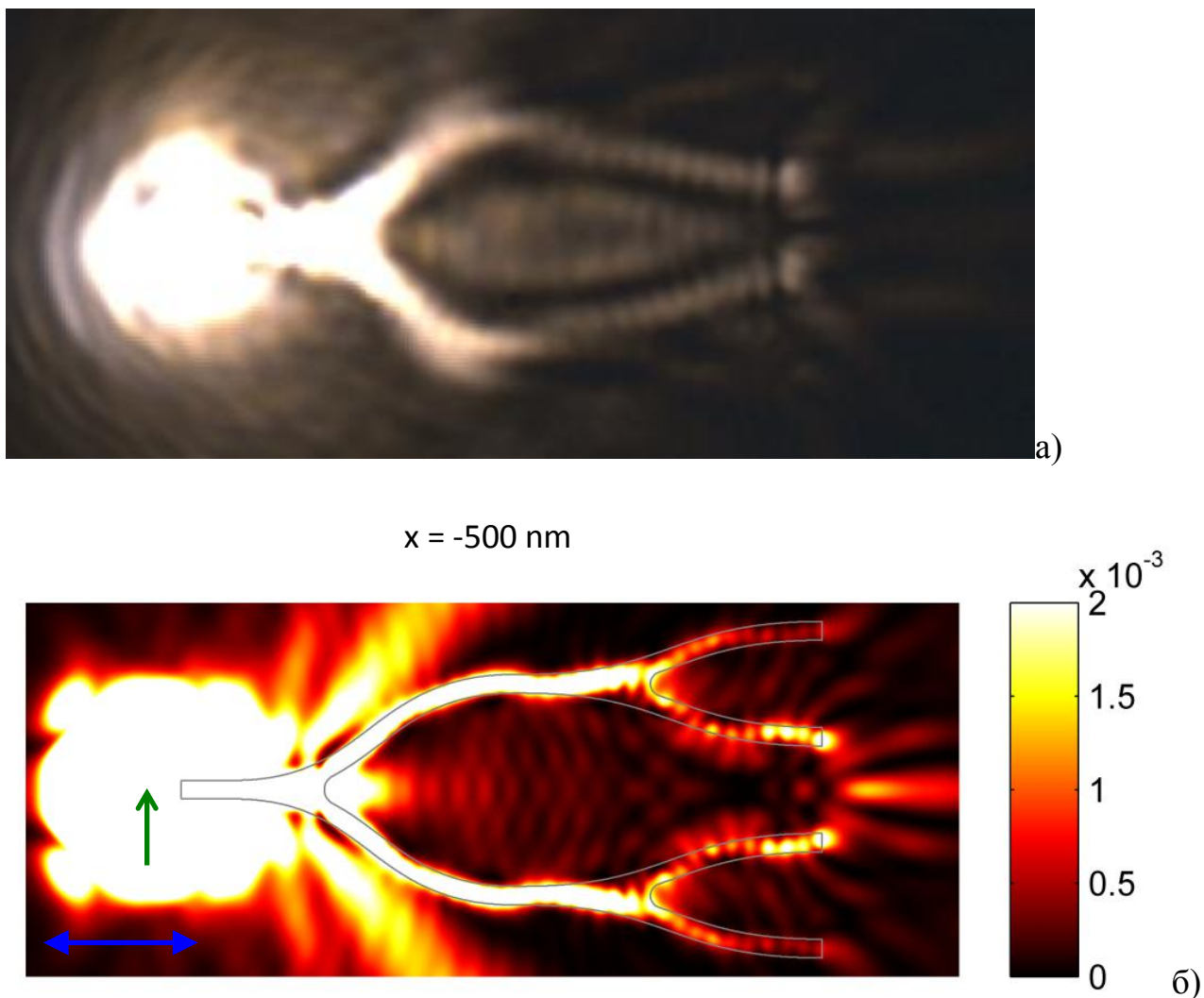
Рисунок 4.7. Поширення ППП у 2-й і 3-й канали розгалужувача (позиція лазерного променя зміщена на -500 \text{ nm} ): а) – експеримент, б) – моделювання.
