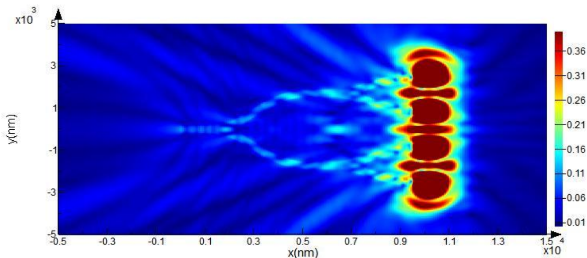
Рис. 2.9. Розподіл інтенсивності поширення ППП по чотирьохканальному мультиплексорі з включенням як суматора (моделювання).
