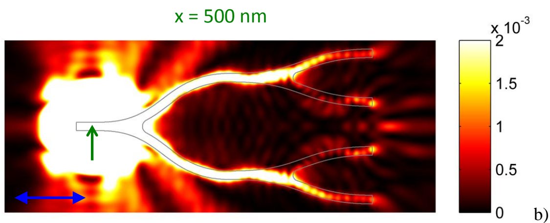
Рисунок 4.8. Поширення ППП у 2 і 3 канали сплітера (позиція лазерного променя зміщена на +500 нм): а) – експеримент, б) – моделювання.
