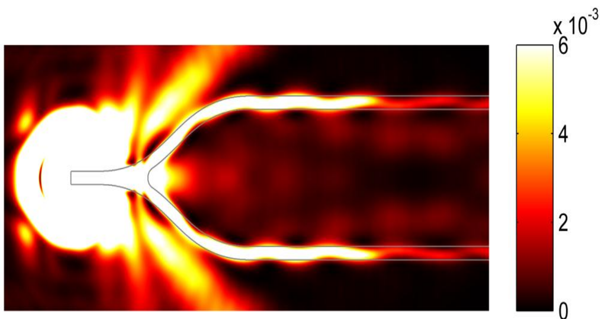
Рис. 3.21. Моделювання поширення ППП у розгалужувачі.
