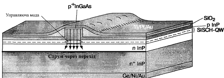
Рис. 1.4. Схема активно-хвилеводної структури з р-n переходом.
