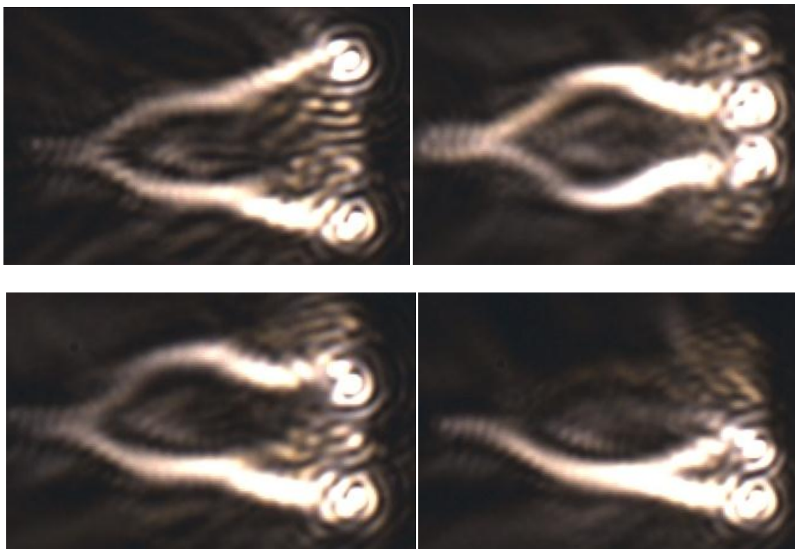
Рисунок 4.14. Поширення ППП у мультиплексорі, включеному як суматор, при використанні двох лазерних променів.
