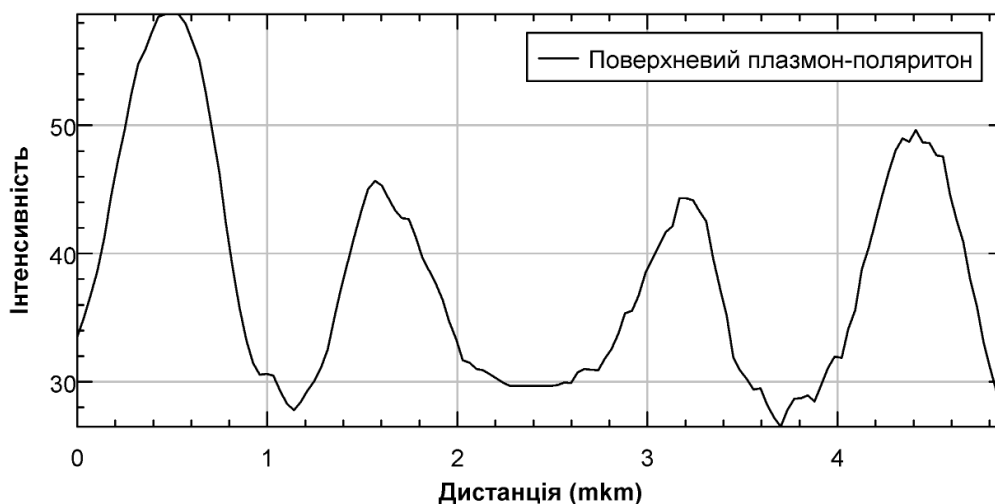
Рисунок 4,3 Інтенсивність ППП на чотирьох виходах розгалужувача.
