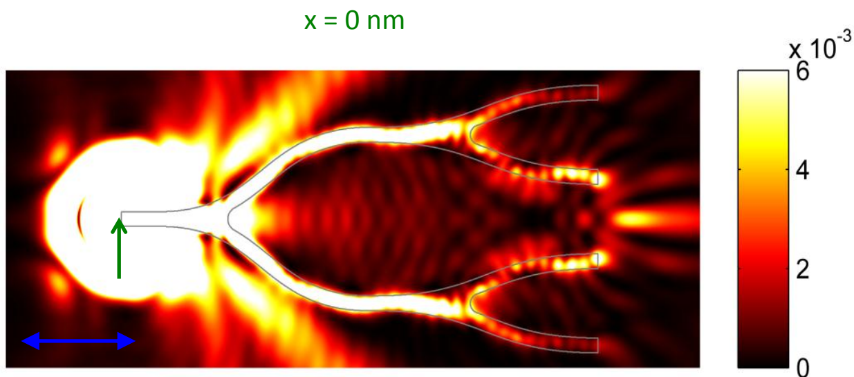
Рис. 2.8 Розподіл інтенсивності поширення ППП по чотирьохканальному мультиплексорі із включенням його як розгалужувача (моделювання).
