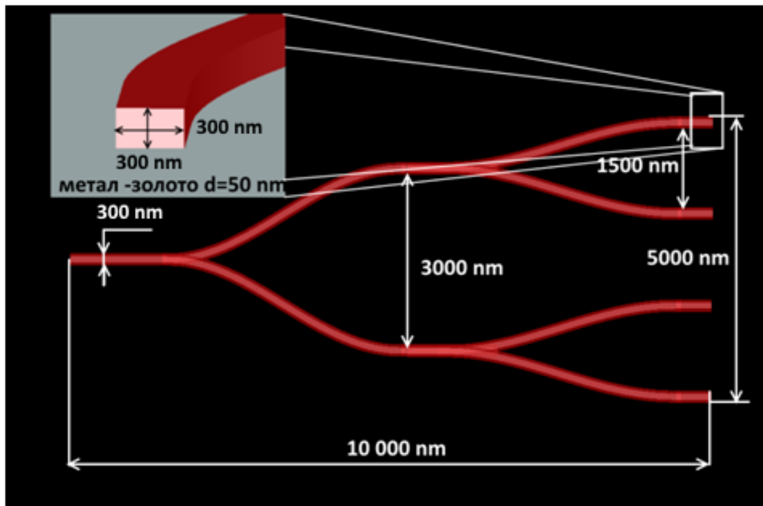
Рис. 2.7. Структурна схема мультиплексора.
