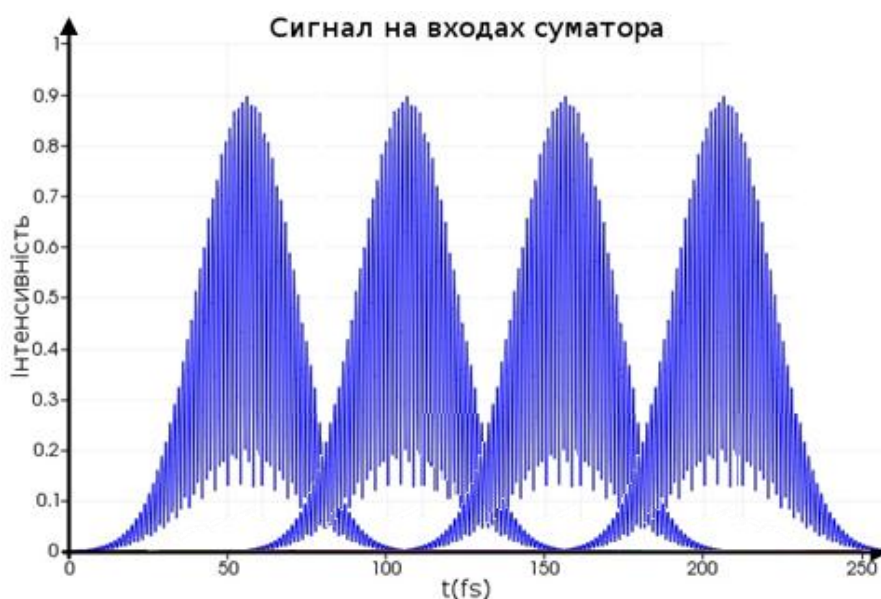
Рис. 2.10 Сигнал, виміряний на вході чотирьохканального суматора, тривалістю 50 фс і віддалю між сигналами 50 фс (моделювання).
