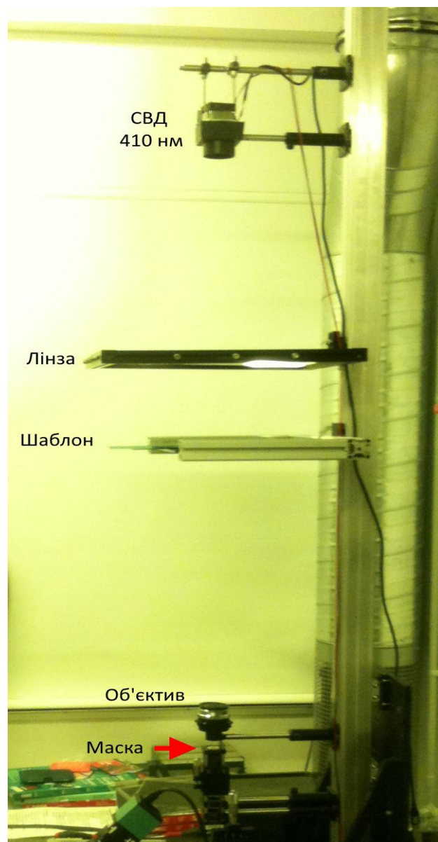
Рисунок 3.6. Технологічна схема процесу зменшення розмірів структур у масштабі 10:1; а) – світло СВД з довжиною хвилі 410 нм; б) – лінза; в) – попередньо підготовлений шаблон діаметром в 20 см; г) – маска діаметром в 2 см [11, 24].
