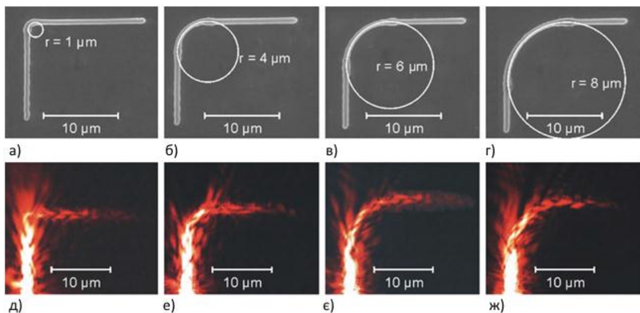
Рисунок 3.14. Поширення ППП при кутах повороту; а – г) – лінійні хвилеводи із зазначеними радіусами кривизни кута повороту, д – ж) – відповідно поширення по цих хвилеводах ППП.
