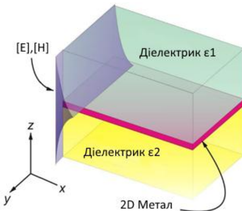
Рис. 2.1. Схематичне зображення структури діелектрик-метал-діелектрик.
