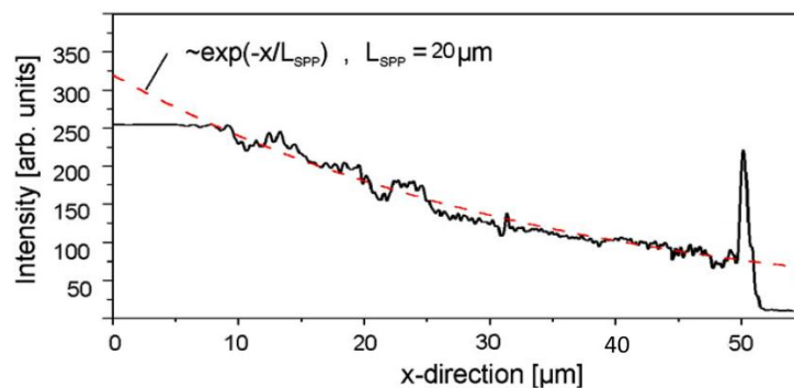
Рис. 3.11. Інтенсивність поширення поверхневого плазмон-поляритону по лінійному хвилеводі довжиною 50 мкм. Суцільна лінія – експериментальний результат, пунктирна лінія – теоретичний розрахунок загасання поверхневого плазмон-поляритону.
