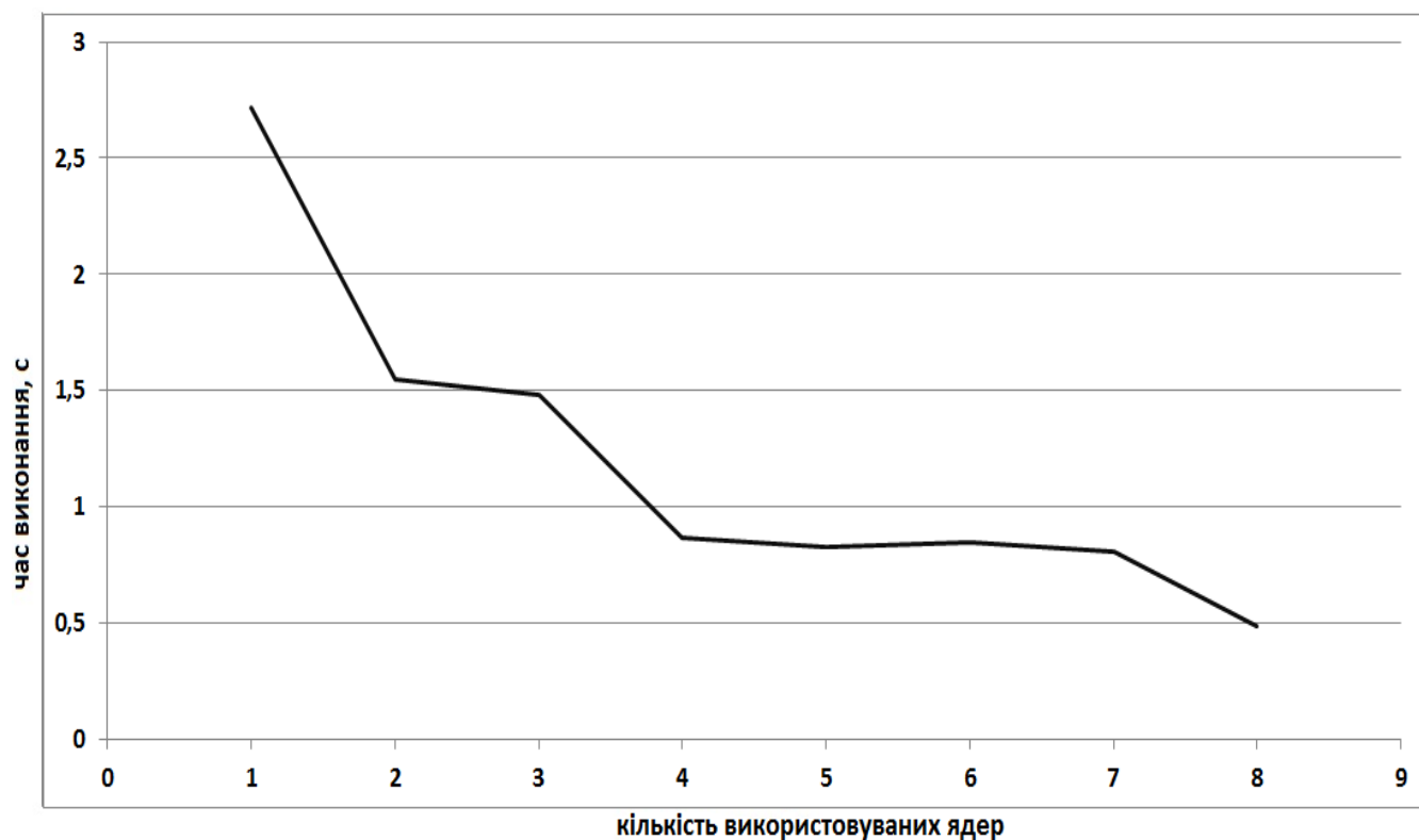
Рис. 4.9. Графік залежності часу виконання від кількості використовуваних ядер
