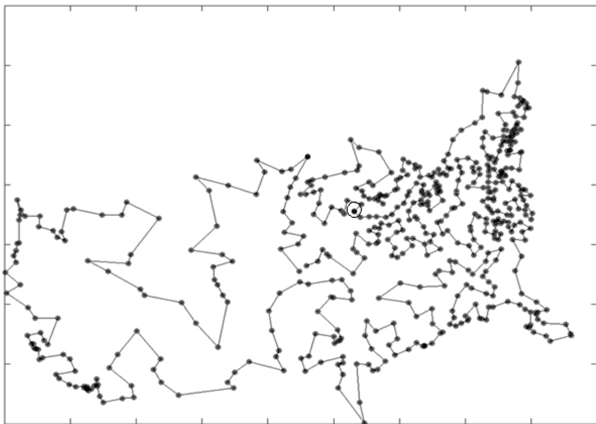
Рис. 4.13. Результуючий маршрут ЗК (АТТ532) отриманий з використанням 3-opt методу локальної оптимізації
