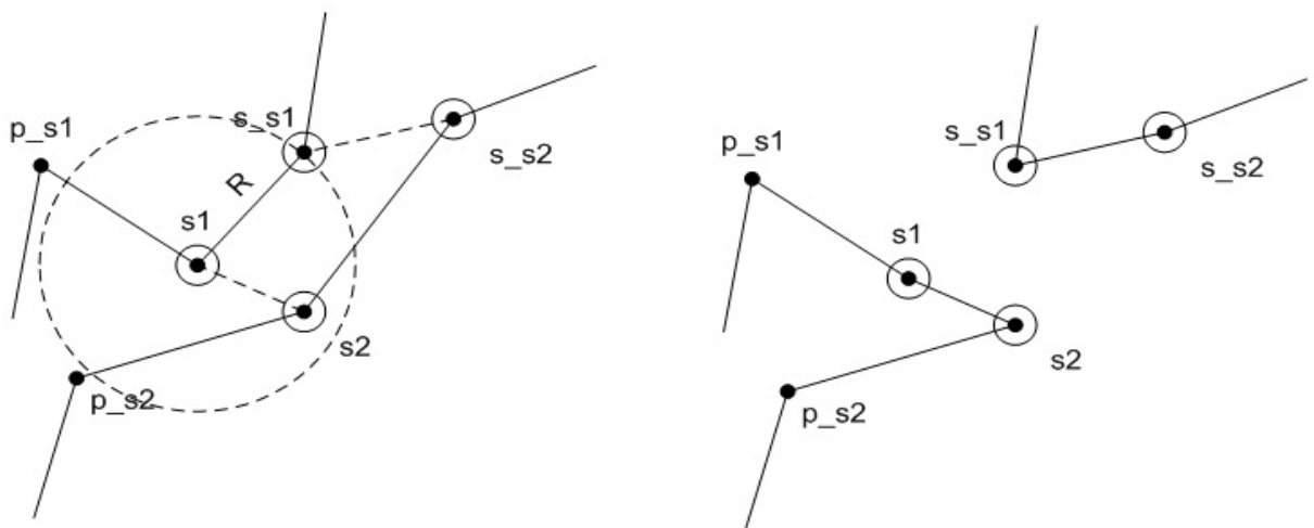
Рис.2.3. Виконання в 2-орт алгоритмі перестановки 1-го типу на довільно обраній ділянці графу
