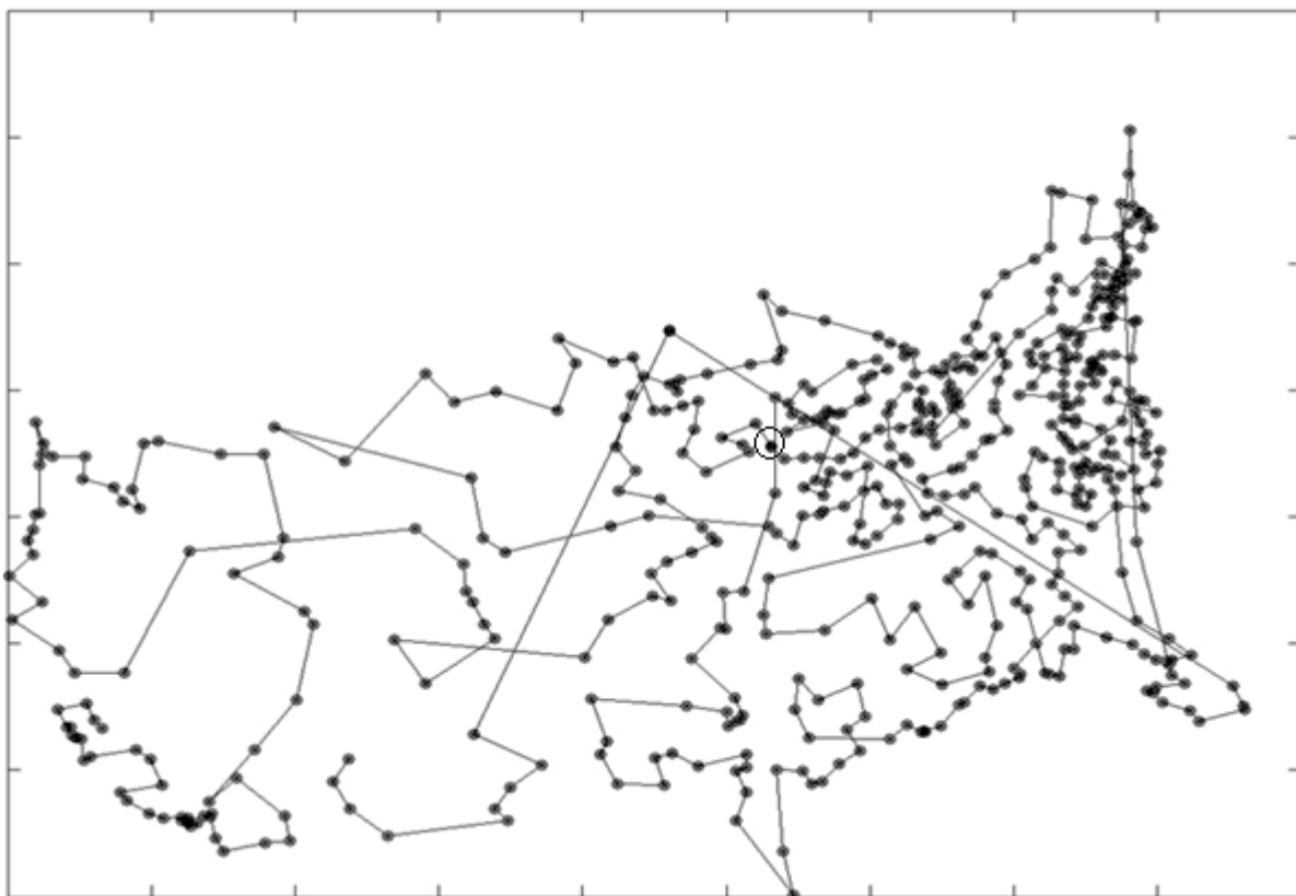
Рис. 4.12. Результуючий маршрут ЗК (АТТ532) отриманий без використання методів локальної оптимізації
