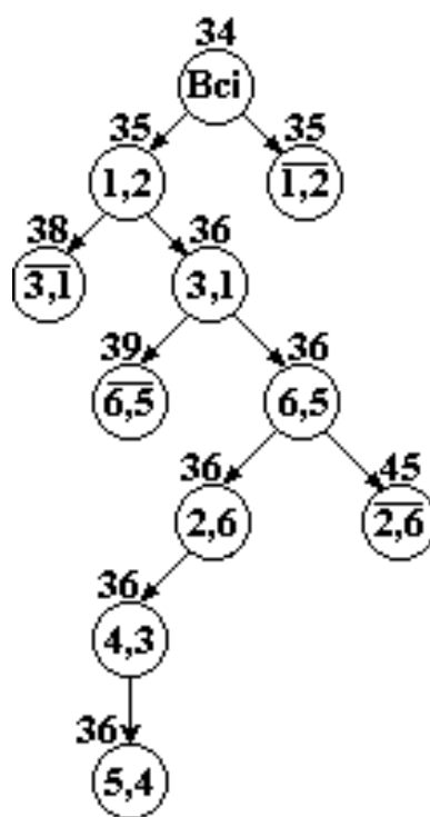
Рис.Е.6. Розв’язок ЗК алгоритмом гілок і меж
