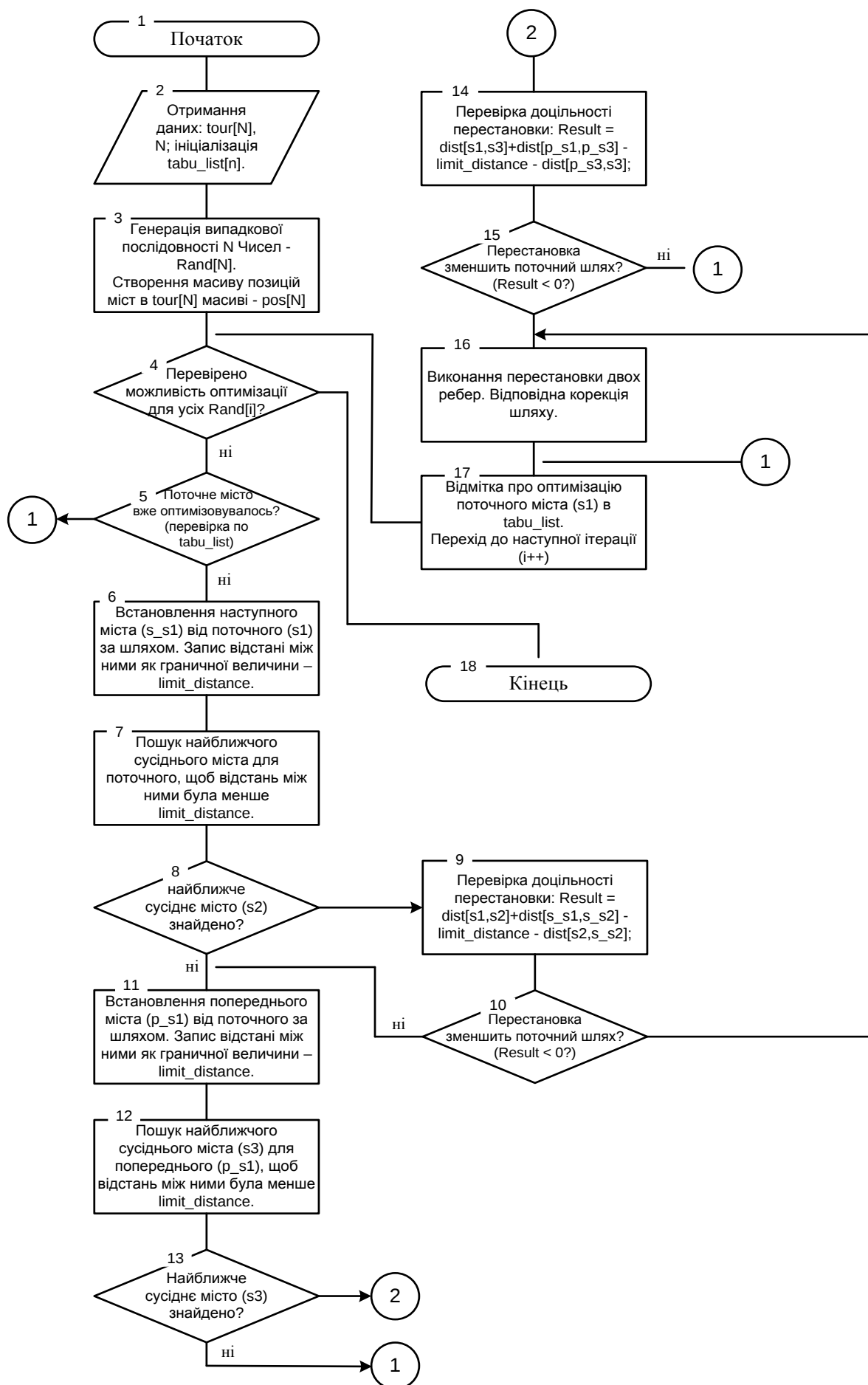
Рис.2.2. Блок-схема програмної реалізації 2-орт алгоритму
