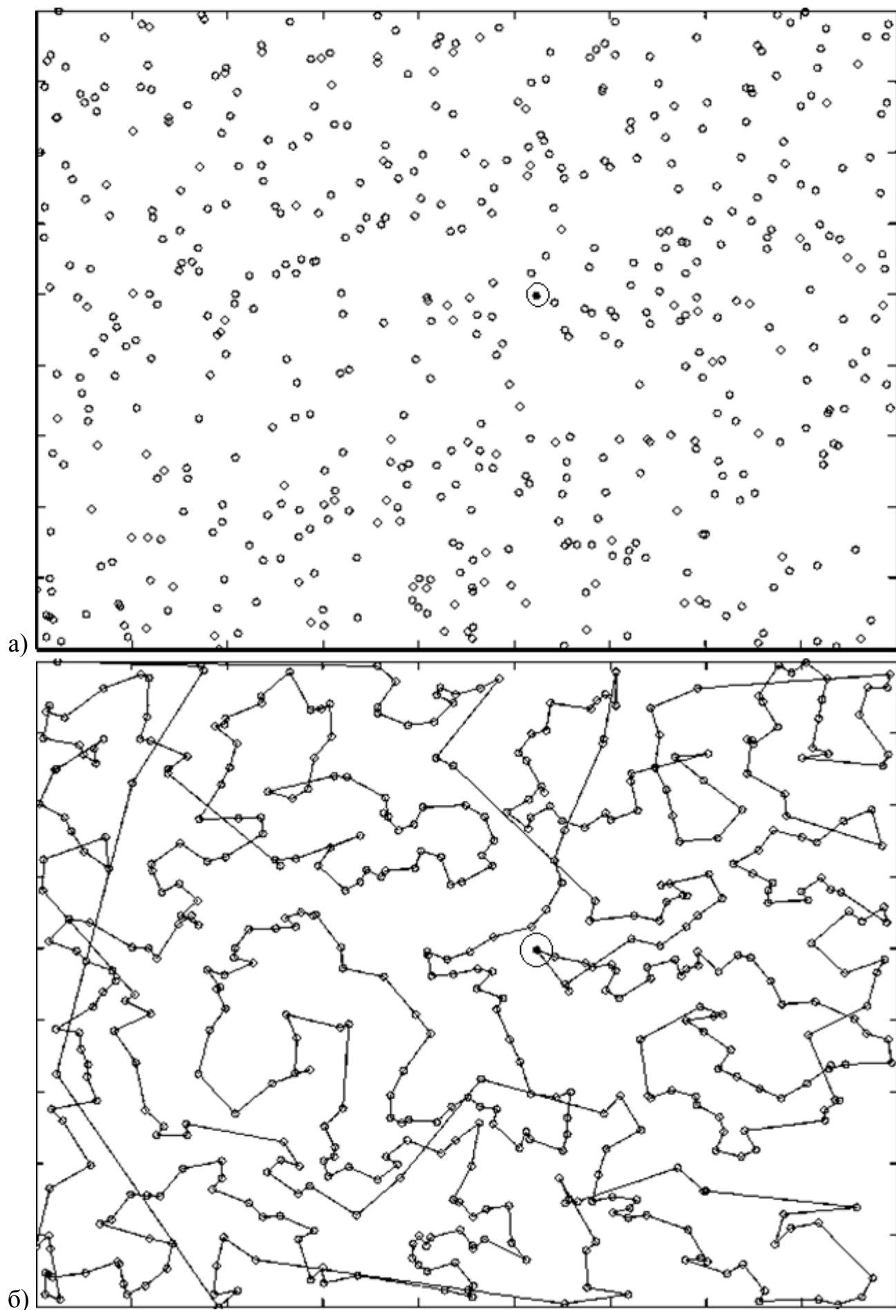
Рис. 4.2. ЗК на 500 вузлів: а) граф вхідної мережі, б) результуючий маршрут
