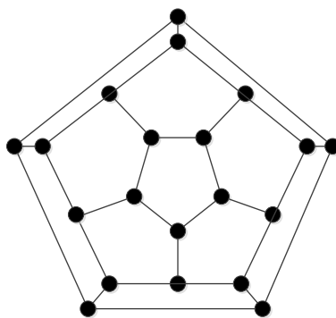
Рис.Д.1. Граф для гри «Кругосвітня подорож»
