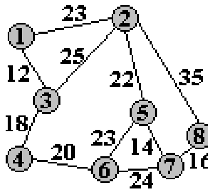
Рис.Е.5. Мережа 3К для алгоритму Дейкстри
