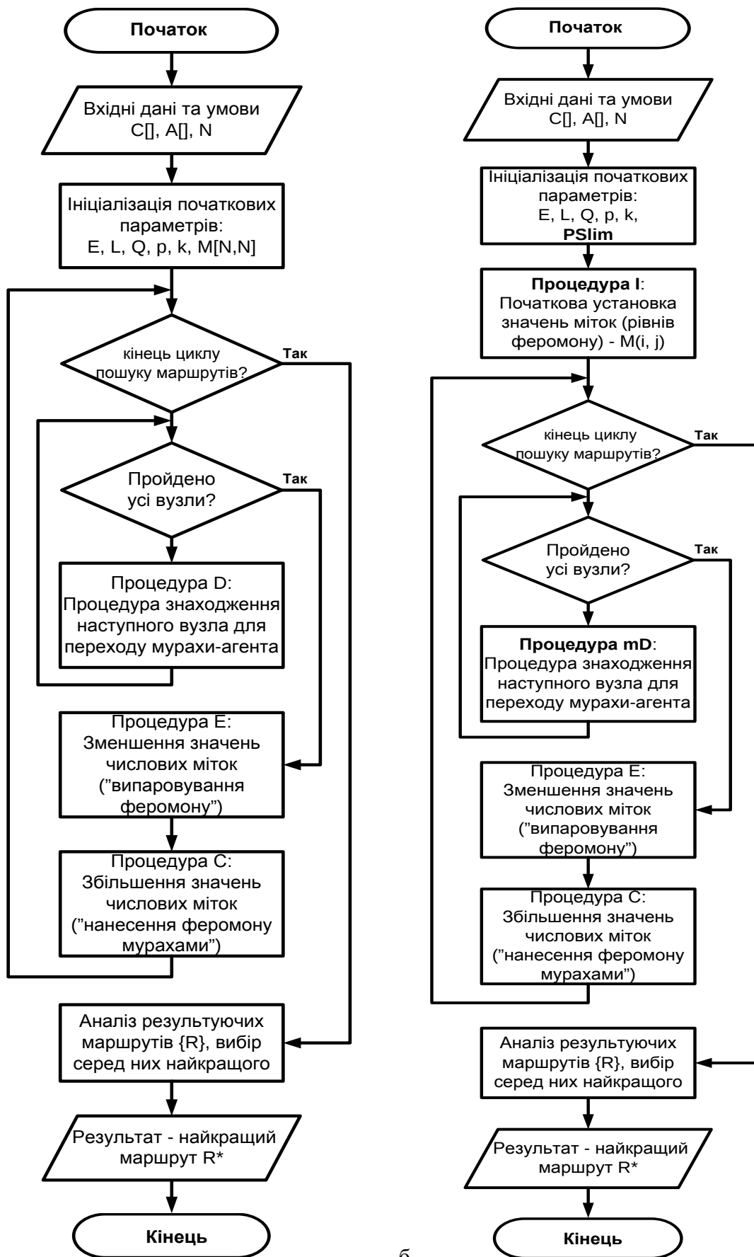
Рис.2.1. Порівняння блок-схем алгоритмів: а) класичний алгоритм колонії мурах, б) алгоритм колонії мурах з врахуванням запропонованої модифікації
